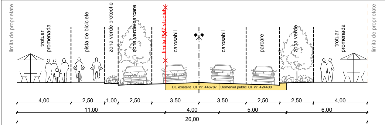
PTT1 - Profil strada colectoare cu infrastructură verde - 26 m - Str. Mitropolit Nicolae Corneanu Extras din Strategia de Dezvoltare Teritorială Urbană - Timișoara Nord, conf. HCL nr. 365/2022
